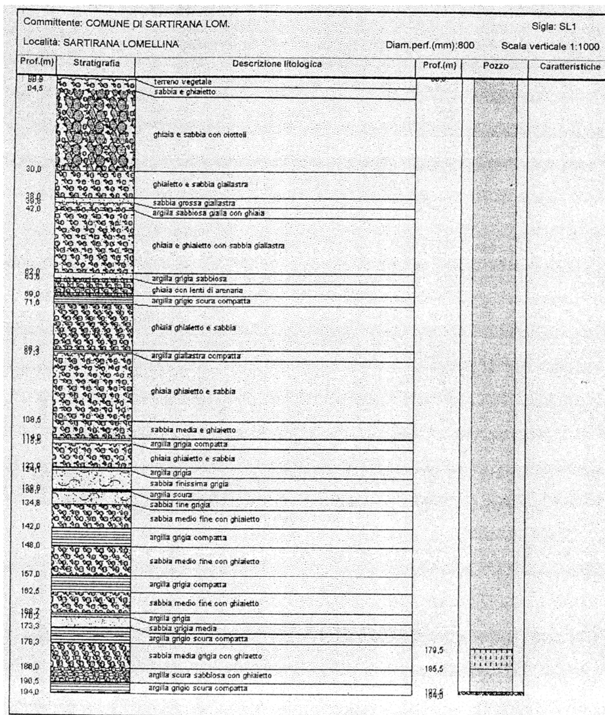
Stratigrafia del pozzo comunale di Sartirana Lomellina
