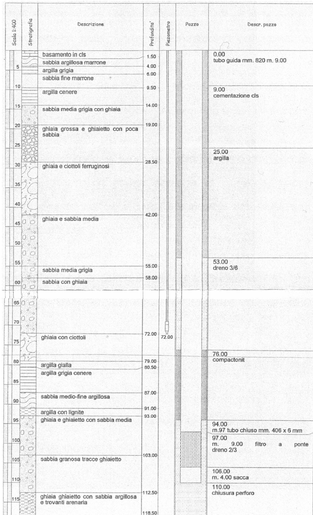
Stratigrafia di un pozzo privato (Ditta Gariboldi)
