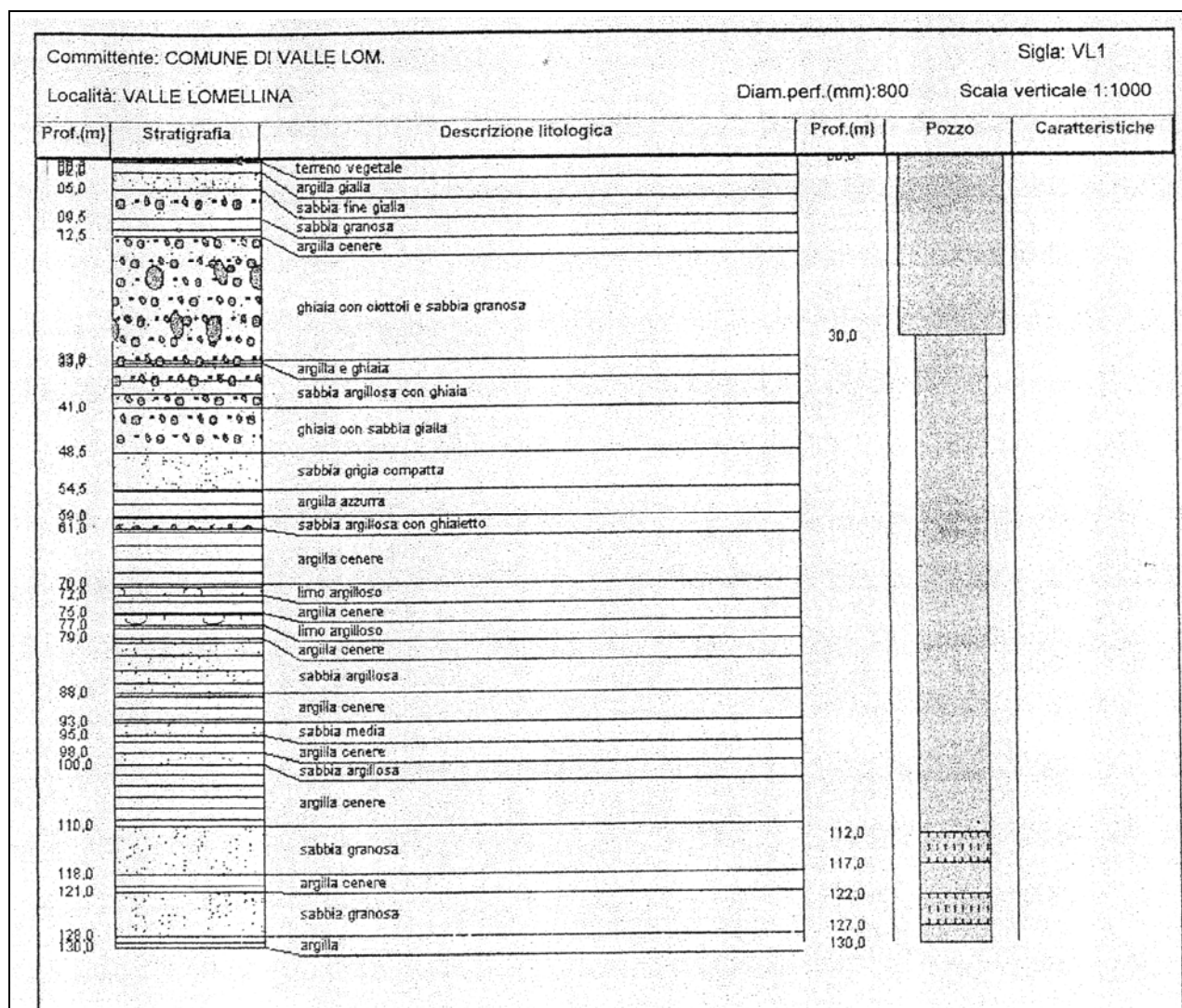
Stratigrafia del pozzo comunale di Valle Lomellina
