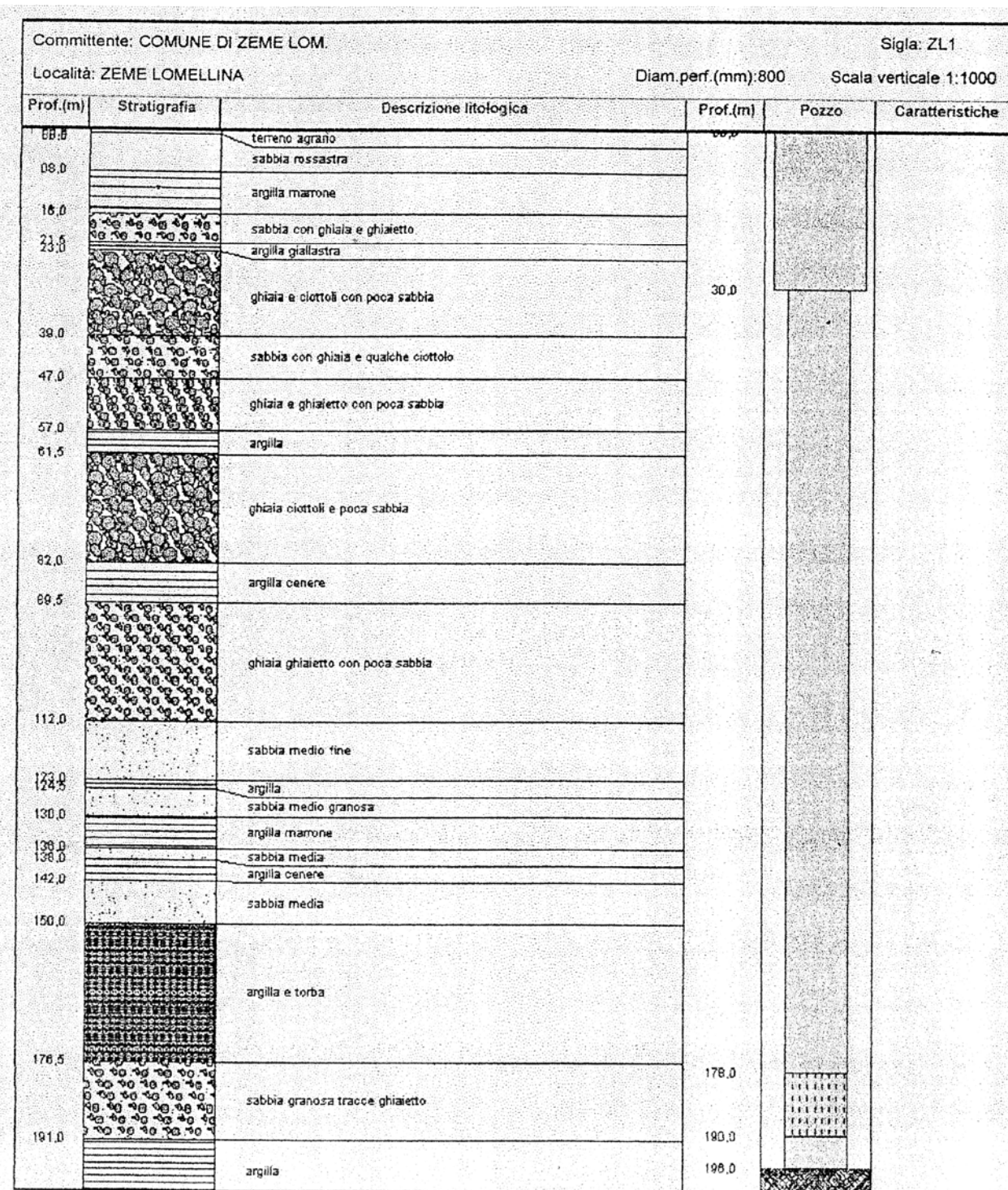
Stratigrafia del pozzo comunale di Zeme Lomellina
